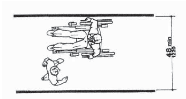
شکل A۱- حداقل عرض گذرگاه برای یک صندلی چرخدار و یک شخص در حال حرکت
