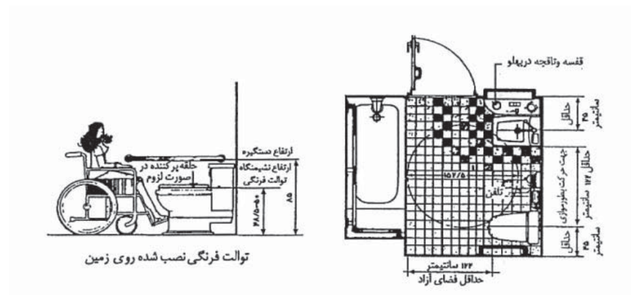
شکل ۲۸- نمونه چیدمان وسایل حمام
