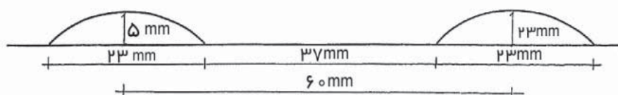
شکل ۴۰- نوع و مشخصات کف پوش پولک دار، ویژه نابینایان
