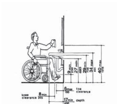
شکل ۳۱- «الف» ابعاد برای نصب دستشویی
