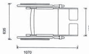
ابعاد ویلچر استاندارد
