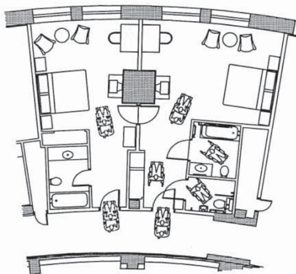
شکل ۵۹- اتاق مهمان قابل دسترسی با سرویس بهداشتی در هتل یا متل
