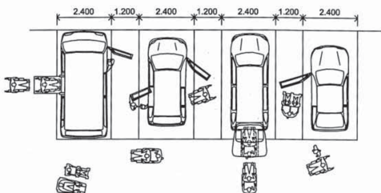
شکل ۱۰-۱۰ (ه) پارکینگ با فاصله مرکزی ۳۶۰۰mm برای افراد دارای معلولیت
