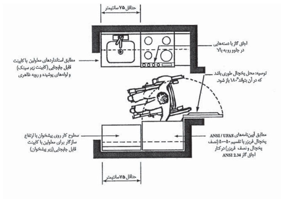
شکل ۳۷- «ب» پلان آشپزخانه کوچک با لوازم سازگار برای معلولین
