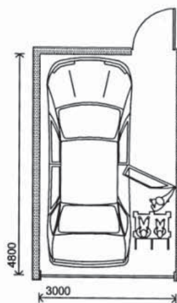
شکل ۱۰-۱۰ (و) پارکینگ ویژه معلولان
