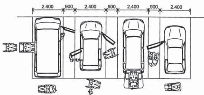
شکل ۱۰-۱۰ (د) پارکینگ با فاصله مرکزی ۳۳۰۰mm برای افراد دارای معلولیت
