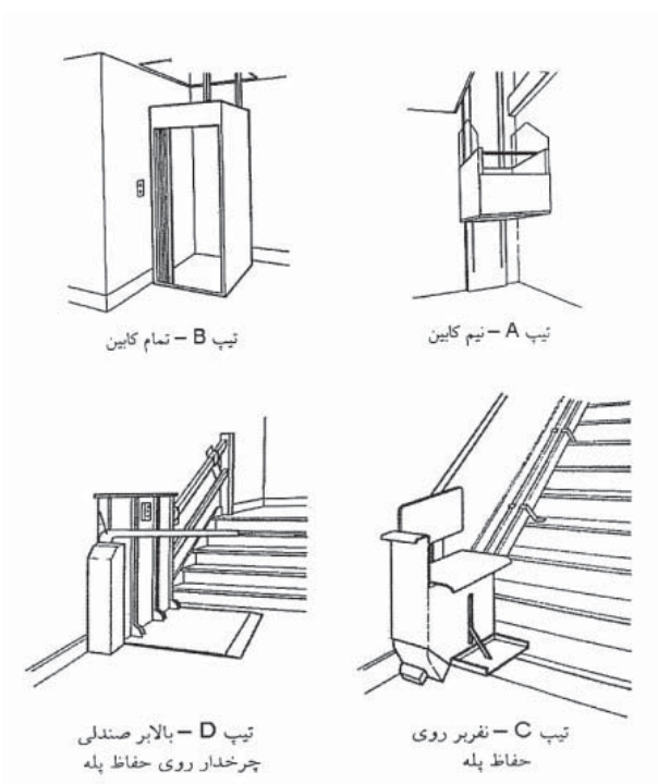
شکل ۲۳- «ج» انواع بالابرهای صندلی چرخدار
